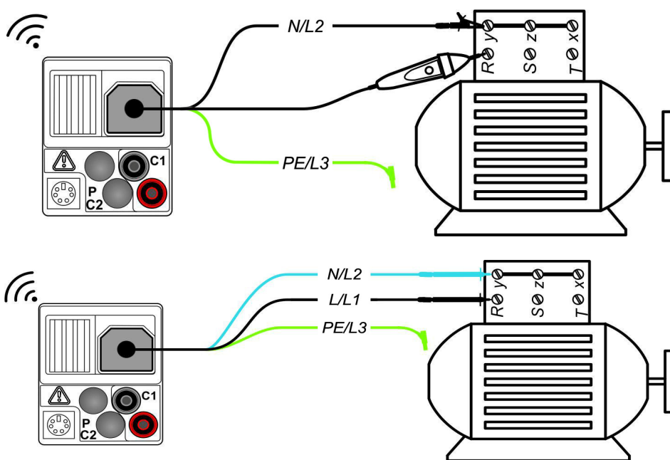
Afbeelding 5.11: Gebruik van de Commander-testpen en 3-geleider testdraad
