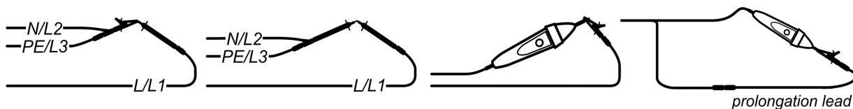
Afbeelding 5.13: Kortgesloten testdraden
