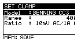
Afbeelding 4.12: Instelling van de stroomtang-meetingang
