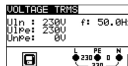
Afbeelding 5.1: Spanning in eenfasestelsel
