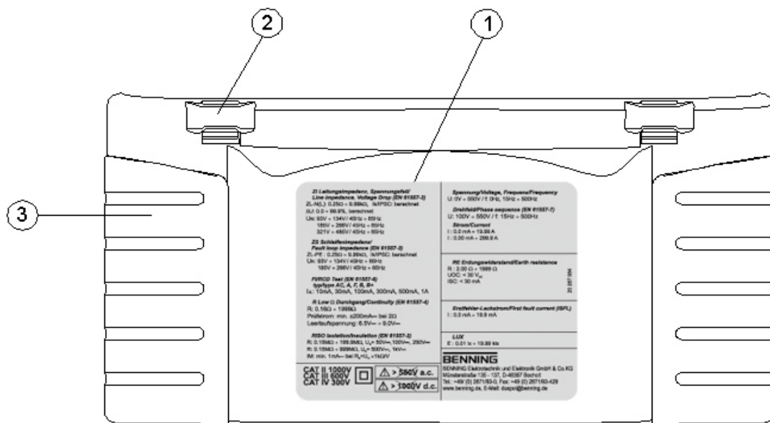
Afbeelding 3.5: Onderaanzicht
