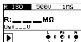
Afbeelding 5.5: Isolati weerstand
