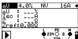
Stap 1 - Zref
