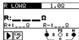
Afbeelding 5.8: Laagohmse weerstand RLOW Ω met 200 mA teststroom
