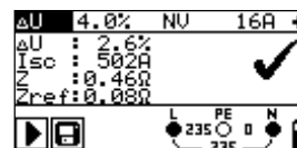
Stap 2 - Spanningsafname
