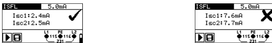
Afbeelding 5.44: Voorbeelden eerstefout-lekstroømmeting
