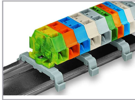
Klemmenstrook; met bevestigingsflenzen; op draagrail 35
