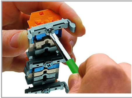
Klemmenstrook; met bevestigingsflenzen,
